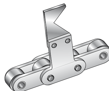
Fig. 21 SA Attachments with Hook
